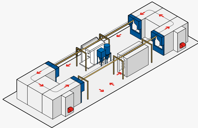
➤ Impianto di verniciatura a polvere automatico
