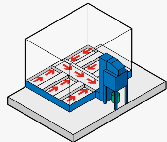
➤ Récupération automatique au-dessus du sol sans génie civil, avec plan de travail surélevé
