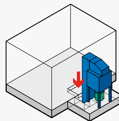
➤ Récupération semi-automatique avec trémie de chargement avec génie civil localisé
